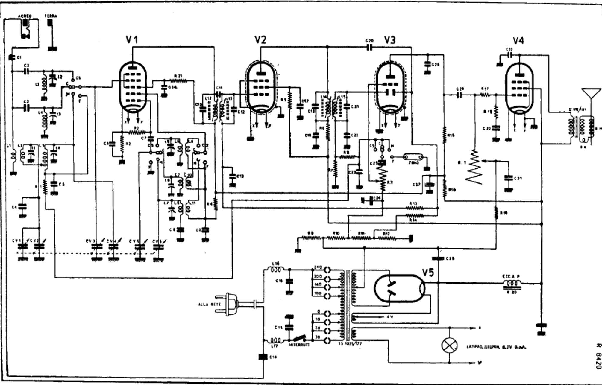
PHONOLA RADIO (S. A. FIMI). — Mod. 561A. — Media frequenza: 470 kHz.
